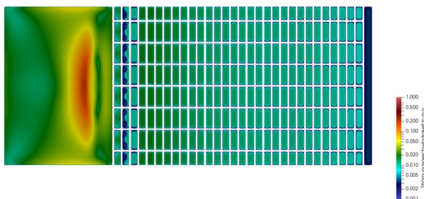
Bild 4 Durchströmung eines mit einem Grobfilter ( k_f = 5 \cdot 10^{-1} \text{ m/s} ) ausgestatteten FiltaPex® · duo 7700 bei einem Zufluss von 45 l/s, Horizontalschnitt durch die Schrägklärereinheit (CFD-Simulation, K.H. Pecher, 2022)
