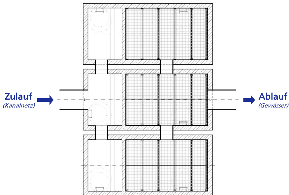
Bild 5 Beispiel für eine Parallelanordnung mehrerer Anlagen vom Typ FiltaPex · duo
