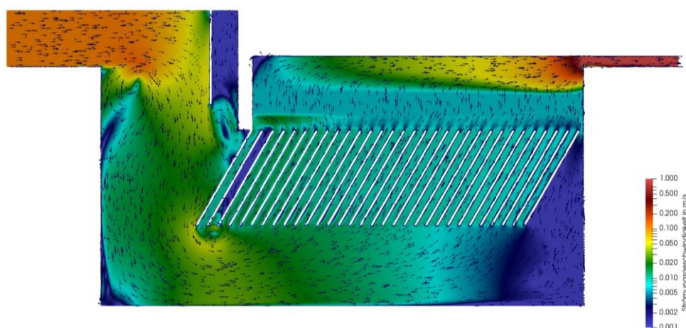
Bild 2 Beispielhafte Durchströmung des FiltaPex® · duo 7700 bei einem Zufluss von 45 l/s und einer Filterdurchlässigkeit von k_f = 2 \cdot 10^{-3} \text{ m/s} (CFD-Simulation, K.H. Pecher, 2022)
