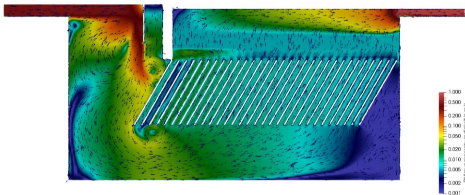
Bild 3 Durchströmung eines mit einem Grobfilter ( k_f = 5 \cdot 10^{-1} \text{ m/s} ) ausgestatteten FiltaPex® · duo 7700 bei einem Zufluss von 45 l/s, Vertikalschnitt in Bauwerksachse (CFD-Simulation, K.H. Pecher, 2022)
